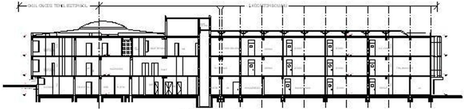
A-A KESİTİ 1/100
