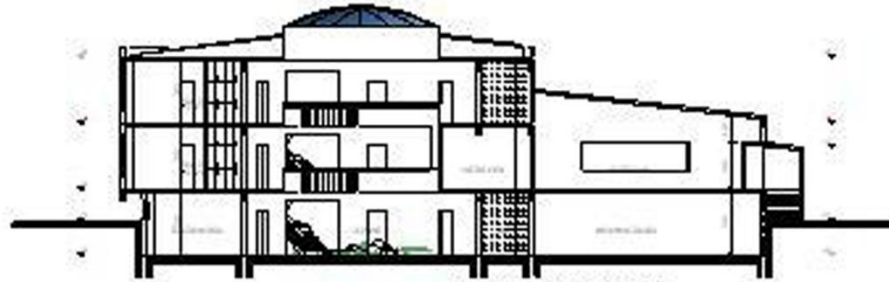
B-B KESİTİ 1/100
