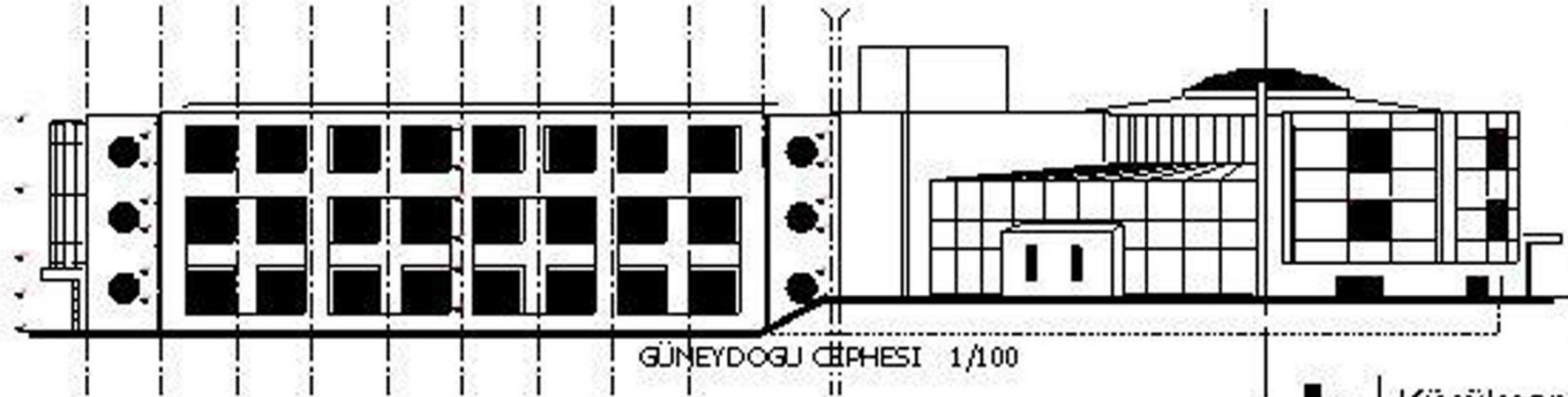
KUZEYDOĞU ÇEŞESİ 1/100
